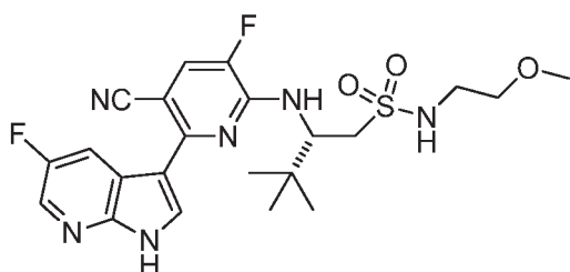
(S)-2-((5-cyano-3-fluoro-6-((S)-2-((5-fluoro-1H-pyrrolo[2,3-b]pyridin-3-yl)pyridin-2-ylamino)-N-(2-methoxyethyl)-3,3-dimethylbutane-1-sulfonamido)-5-fluoro-1H-pyrrolo[2,3-b]pyridin-3-yl)pyridin-2-ylamino)-N-(2-methoxyethyl)-3,3-dimethylbutane-1-sulfonamide (29)
