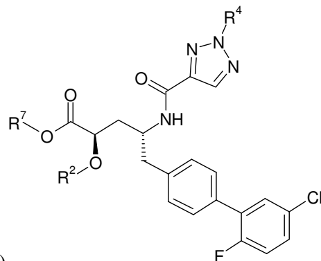
(VIIIb)
