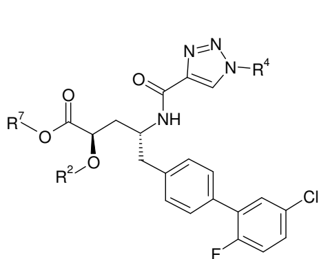
(VIIIa)
