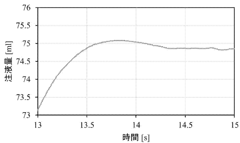
(2) 拡大図 (注液ポート内径=4mm)
