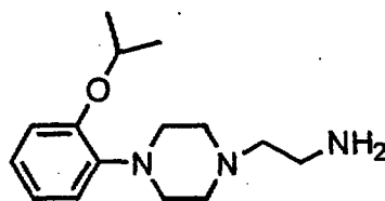
Cpd. 2
