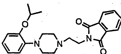
Cpd. 1
