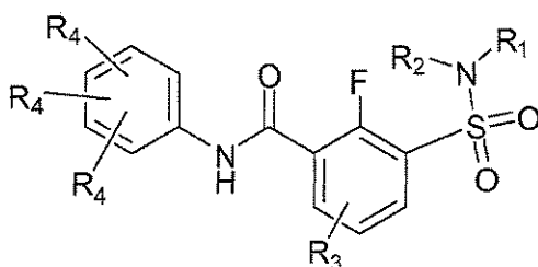
(Id)
