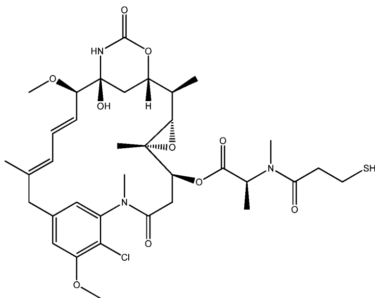
Mertansine (DM1)
