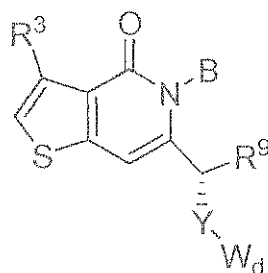
Formula (IX).
