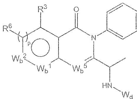
(XXII).
