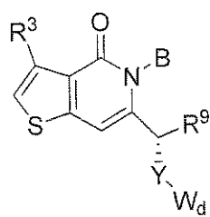
Formula (IX).
