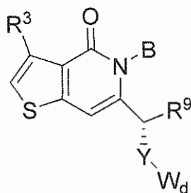
Formula (IX).
