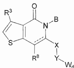
Formula (VI);
