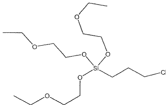
3-Chloropropyltri(2-ethoxyethoxy)silane
