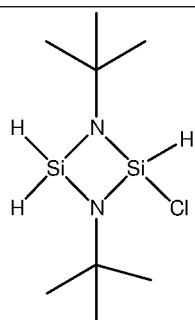
1,3-bis(tert-butyl)-2-chlorocyclodisilazane
