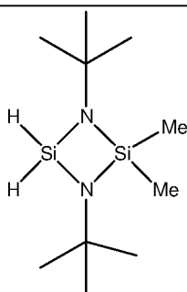
1,3-bis(tert-butyl)-2- dimethylcyclodisilazane
