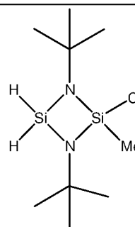
1,3-bis(tert-butyl)-2-chloro-2- methylcyclodisilazane
