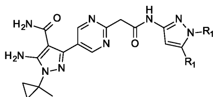
III m ,
