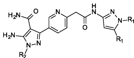
Ie,
