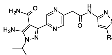
IIv,
