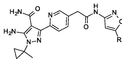
IIIg,
