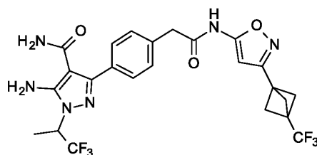
Example 259
