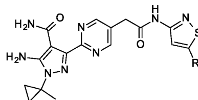
IIIr,
