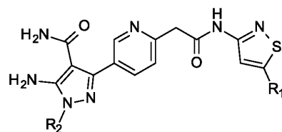
If,
