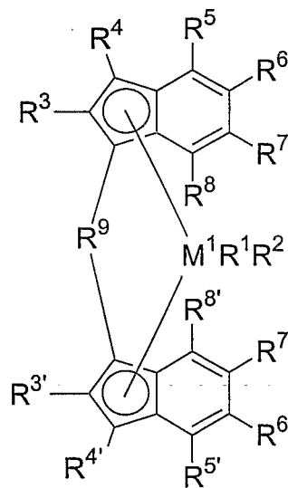
meso/pseudomeso isomer
