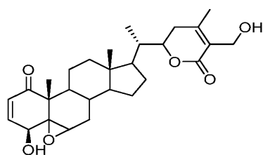
Withaferin-A
