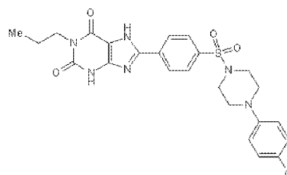
PSB-603
