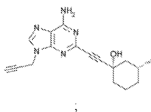
ATL-444
