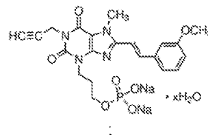
MSX-3
