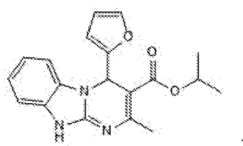
PSB-1115
