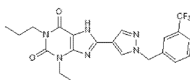
PSB-0788
