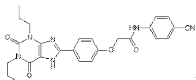
ISAM-140
