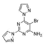
PBF-509 (NIR178)
