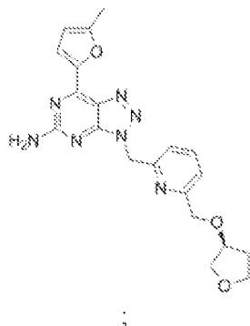
PBF-509 (NIR178)
