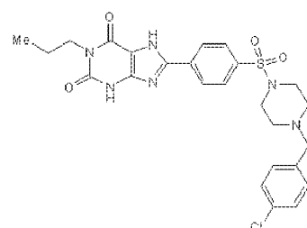
PSB-603
