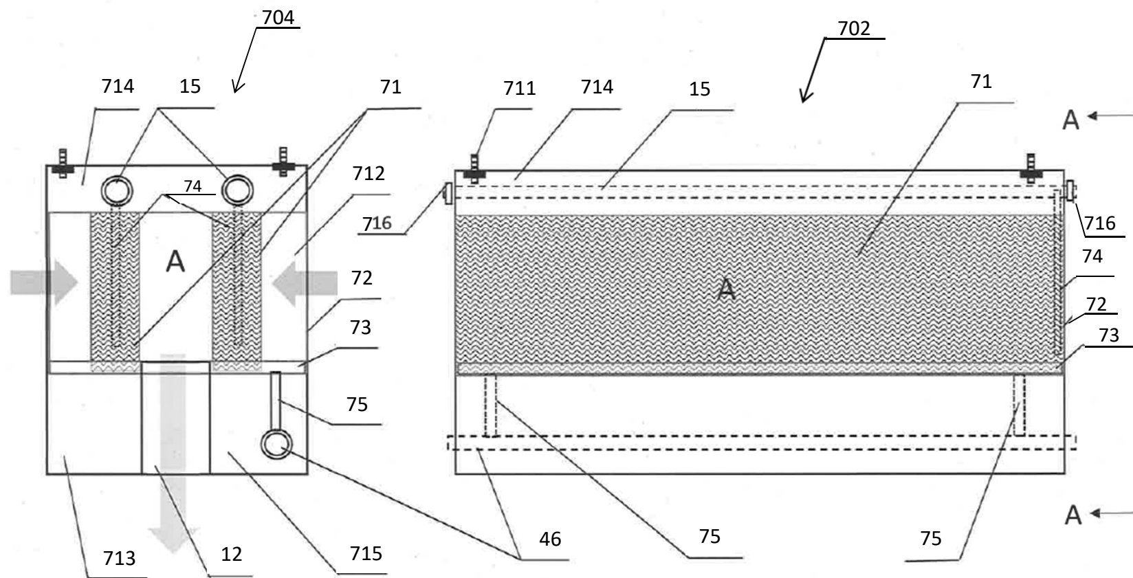
Section A-A
