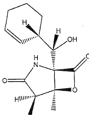
II-20
