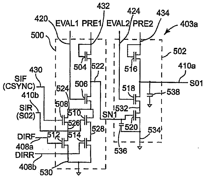
Fig. 10A
