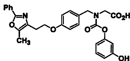
Example 308
