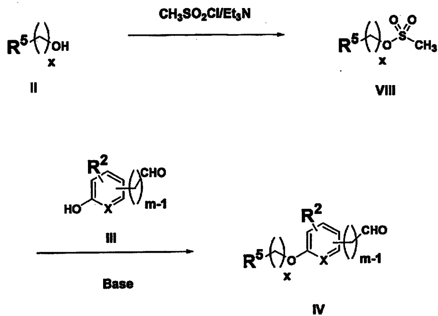
SCHEME 1A
