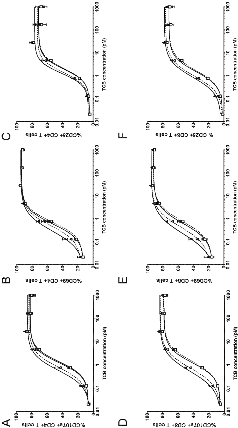
▲ CD19(2B11) CD3opt ■ CD19(2B11) CD3orig △ CD19(018) CD3opt □ CD19(018) CD3orig FIG. 9
