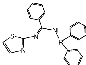
NP Amidine XXVII
