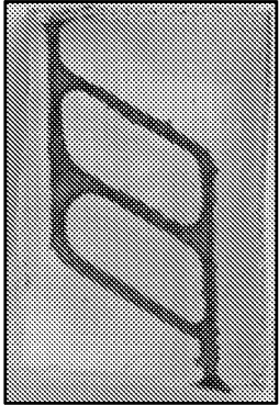
PDMS
