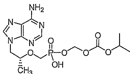
mono-POC PMPA
