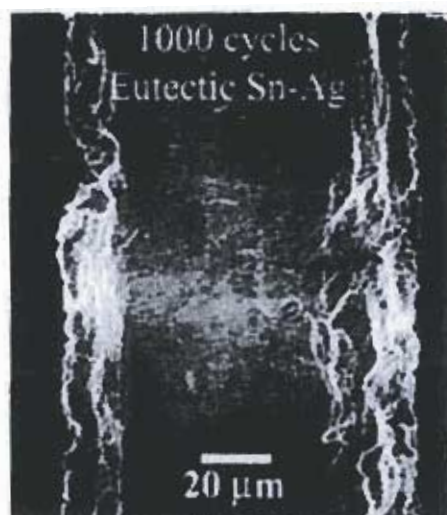
Fig. 47A eutectic Sn-Ag
