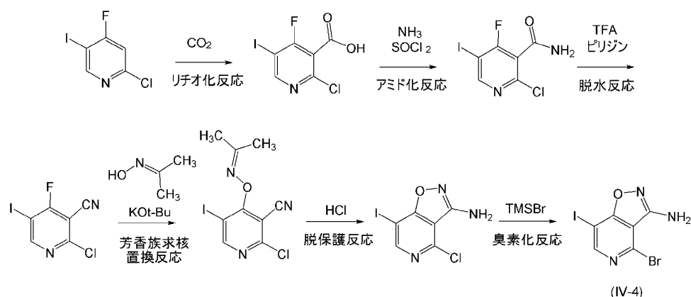
反応工程式 2
