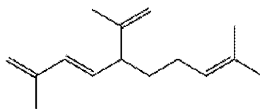
(E)-2,9-dimethyl-5-(prop-1-en-2-yl)deca-1,3,8-triene
