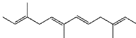
(2E,5E,7E,10E)-3,6,10-trimethyldodeca-2,5,7,10-tetraene
