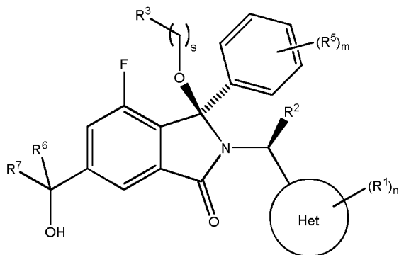
Diastereoisomer 1A
