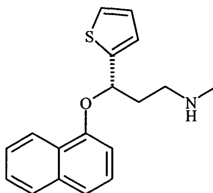
( S )-duloxetine
