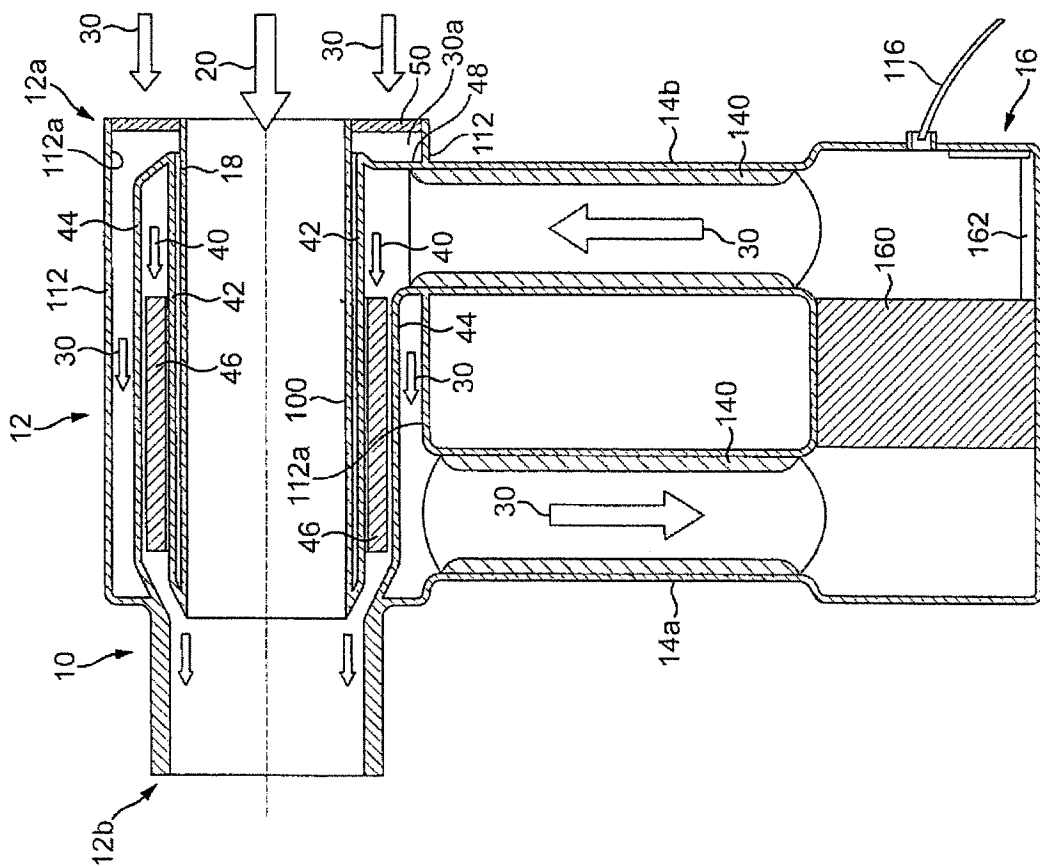
M - M FIG. 8
