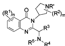
(IVa)
