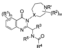
(IIIb)
