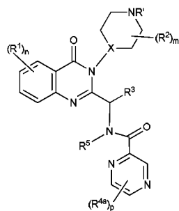
(IIId)
