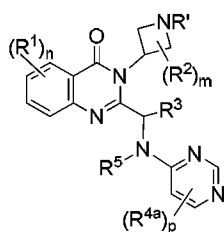
(Va)
