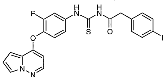
1-(4-( H -Pyrrolo[1,2- b ]pyridazin-4-yloxy)-3-fluorophenyl)-3-(2-(4-fluorophenyl)acetyl)thiourea
