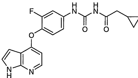
1-(4-(1H-Pyrrolo[2,3-b]pyridin-4-yloxy)-3-fluorophenyl)-3-(2-cyclopropylacetyl)urea
