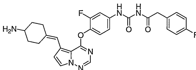
1-(4-(5-((4-Aminocyclohexylidene)methyl)pyrrolo[2,1- f ][1,2,4]triazin-4-yloxy)-3-fluorophenyl)-3-(2-(4-fluorophenyl)acetyl)urea
