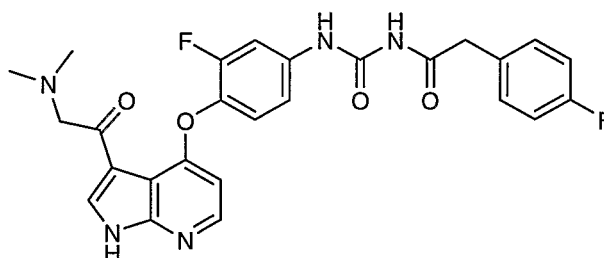
1-(4-(3-(2-(Dimethylamino)acetyl)-1H-pyrrolo[2,3-b]pyridin-4-yloxy)-3-fluorophenyl)-3-(2-(4-fluorophenyl)acetyl)urea
