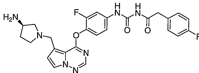
(R)-1-(4-(5-((3-Aminopyrrolidin-1-yl)methyl)pyrrolo[2,1-f][1,2,4]triazin-4-yloxy)-3-fluorophenyl)-3-(2-(4-fluorophenyl)acetyl)urea
