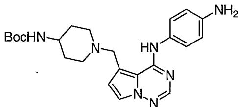
1-(4-(5-((4-Aminopiperidin-1-yl)methyl)pyrrolo[2,1-f][1,2,4]triazin-4-ylamino)phenyl)-3-(2-(4-fluorophenyl)acetyl)urea
