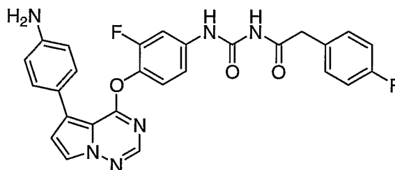
1-(4-(5-(4-Aminophenyl)pyrrolo[2,1-f][1,2,4]triazin-4-yloxy)-3-fluorophenyl)-3-(2-(4-fluorophenyl)acetyl)urea
