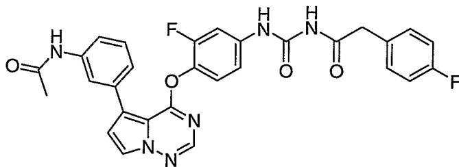
1-(4-(5-(3-Acetamidophenyl)pyrrolo[2,1-f][1,2,4]triazin-4-yloxy)-3-fluorophenyl)-3-(2-(4-fluorophenyl)acetyl)urea
