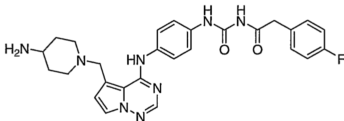
1-(4-(5-((4-Aminopiperidin-1-yl)methyl)pyrrolo[2,1-f][1,2,4]triazin-4-ylamino)phenyl)-3-(2-(4-fluorophenyl)acetyl)urea
