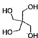
pentaerythritol
