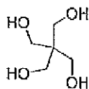
pentaerythritol
