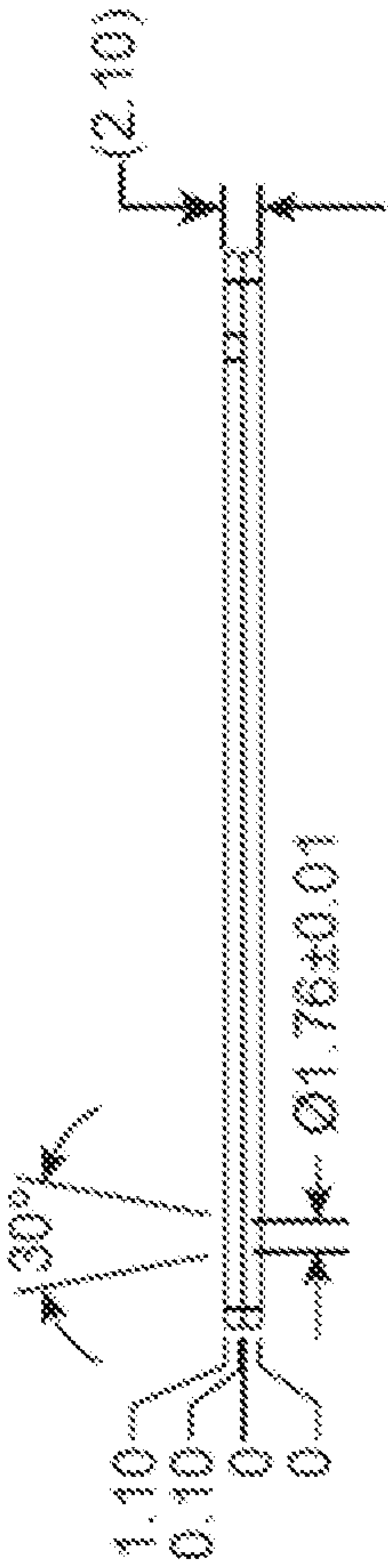
SECTION A-A
