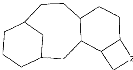
(XXIX)
