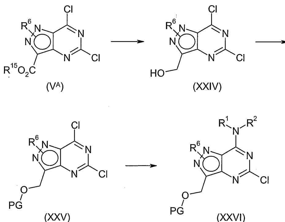
Scheme 25A
