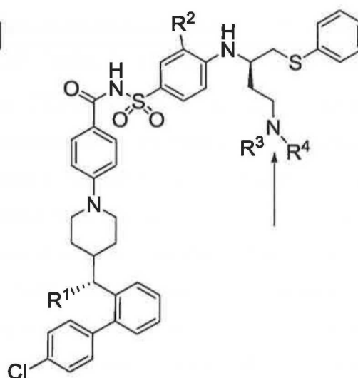
Formula (I-b)
