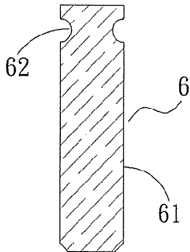
A-A FIG. 2 PRIOR ART
