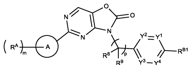
Formula (IIb-1a).
