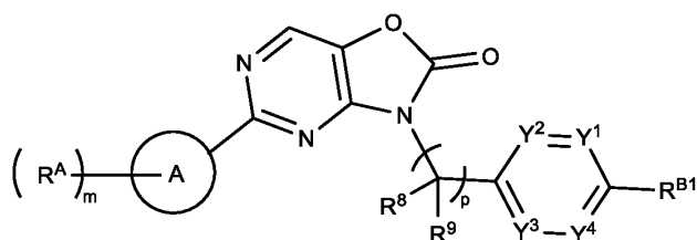
Formula (IIb-1a).
