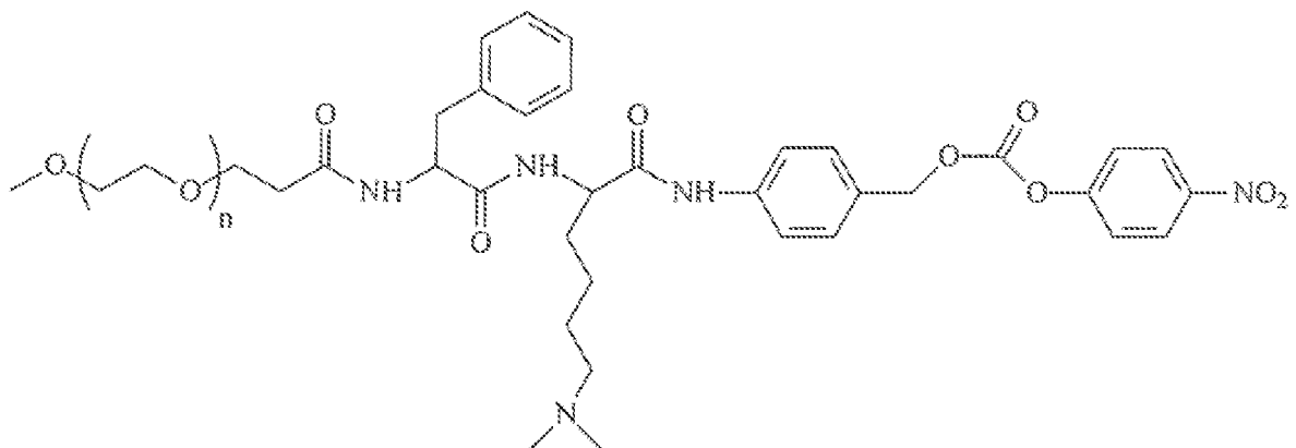
PEG-PheLys(CH 2 ) 2 -PABC-PNP
