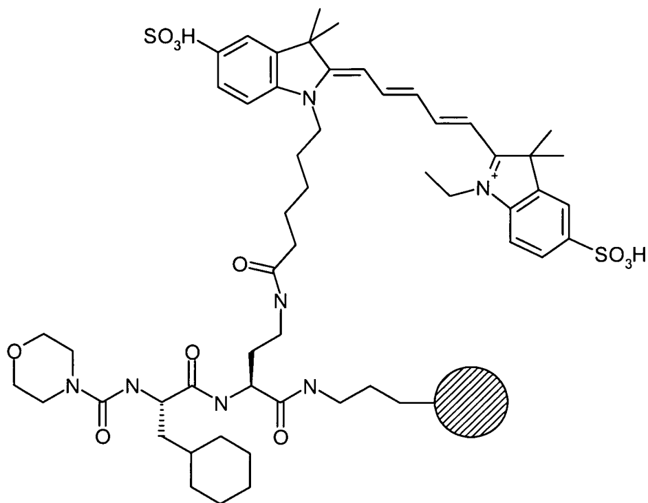
(Scheme 15).
