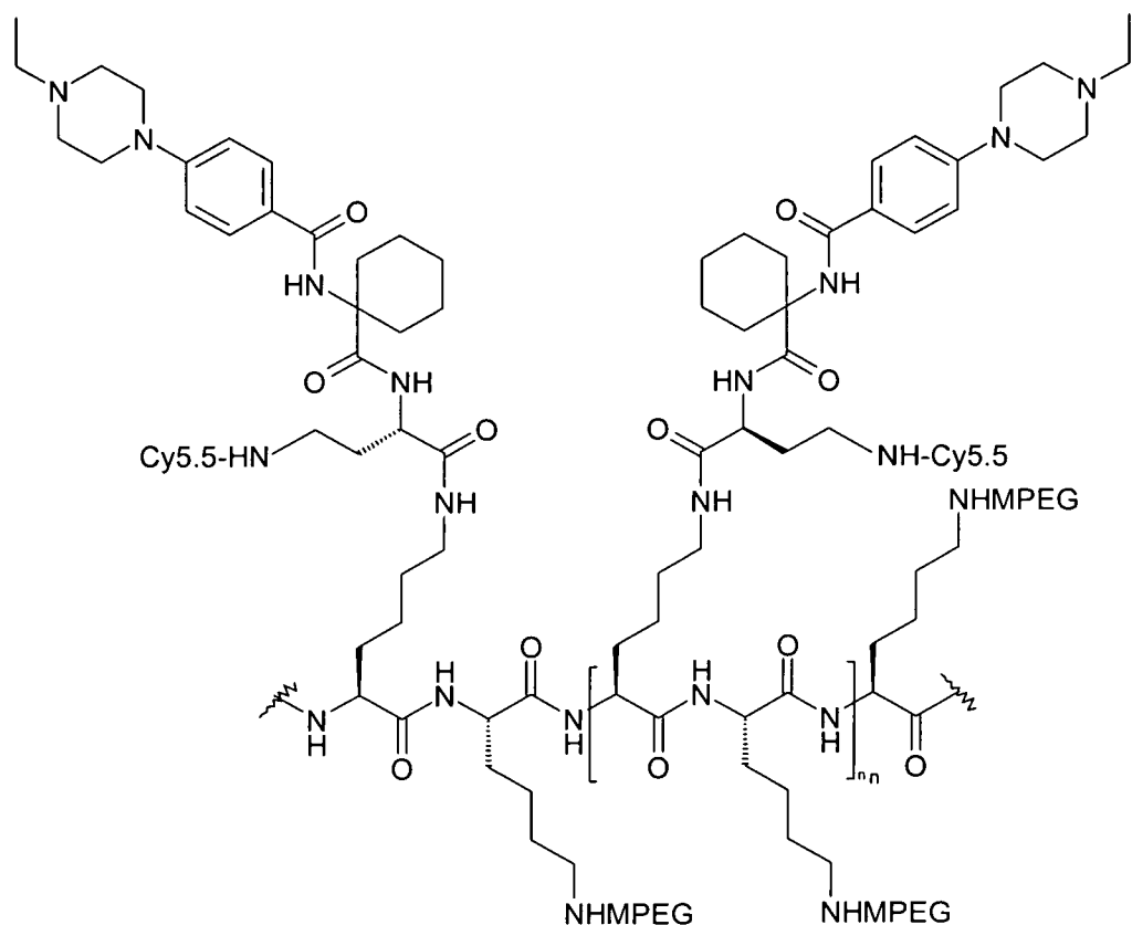
(Scheme 20)
