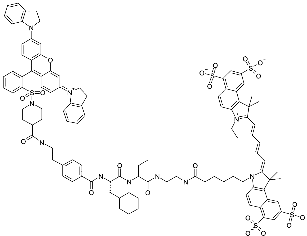
(Scheme 5)
