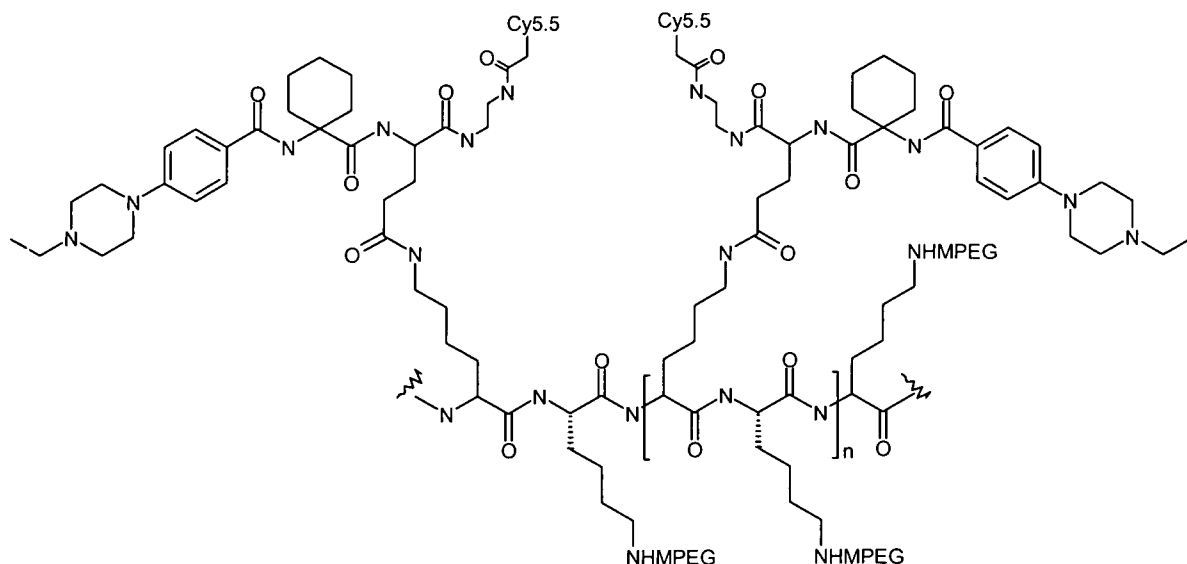
(Scheme 19)
