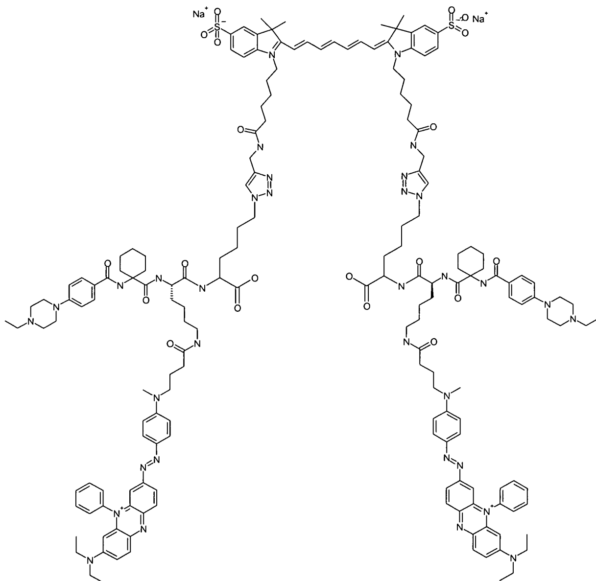
(Scheme 18).
