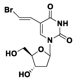
Brivudine (BVDU)
