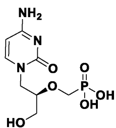
Cidofovir (CDV)
