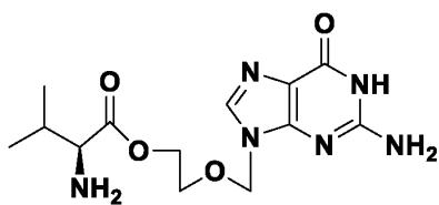
Valacyclovir (VACV)
