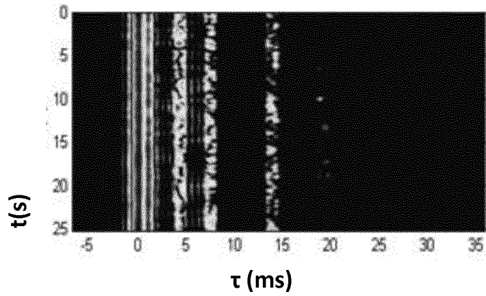
Réponse d'impulsion de canal en bande limitée
