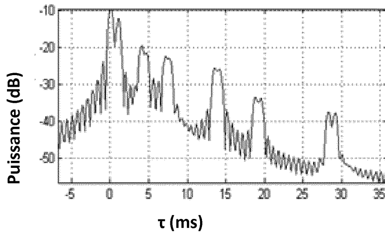
Profil de retard en puissance en bande limitée
