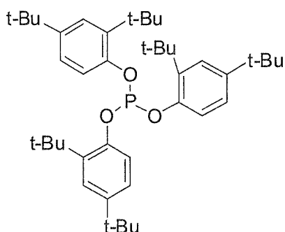
Tris(2,4-di-tert-butylphenyl)phosphite (TDTBPP)
