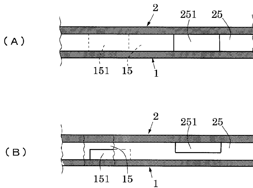
図5の矢視N
