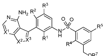
Formula I-A
