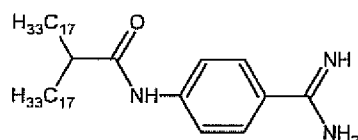
BADACA (Benzamindin-DACA)
