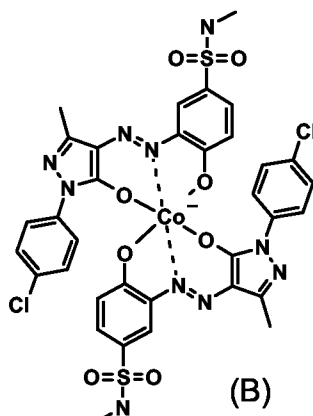
Azo metal Complex B
