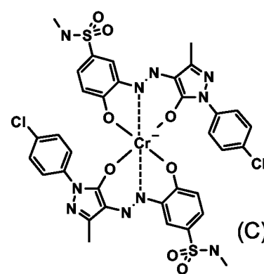
Azo metal Complex C
