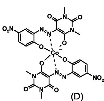
Azo metal Complex D
