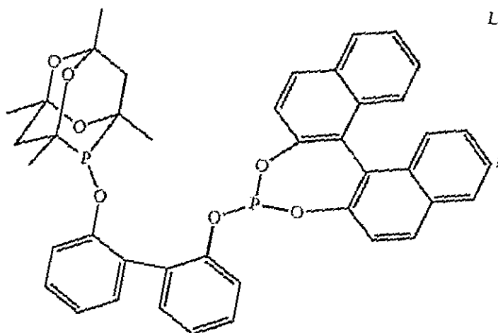
Ligand E
