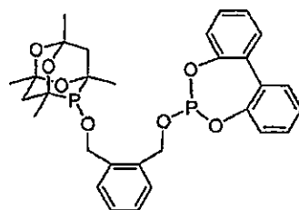
Ligand B
