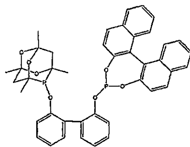
Ligand D
