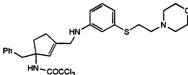
Cpd. 21
