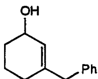
Cpd. 2
