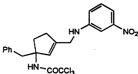
Cpd. 23
