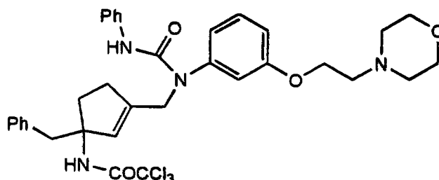
Cpd. 7
