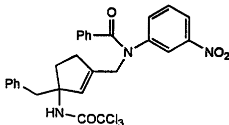
Cpd. 24
