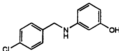
Cpd. 27
