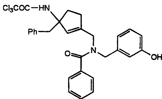
Cpd. 31
