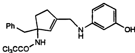
Cpd. 42
