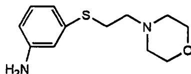
Cpd. 20
