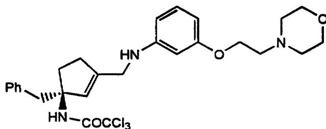
Cpd. 6a
