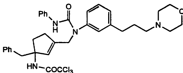
Cpd. 19
