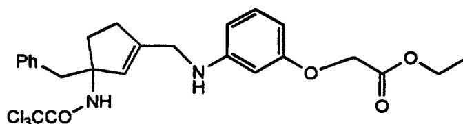
Cpd. 43
