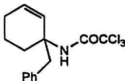
Cpd. 3
