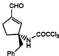
Cpd. 4b
