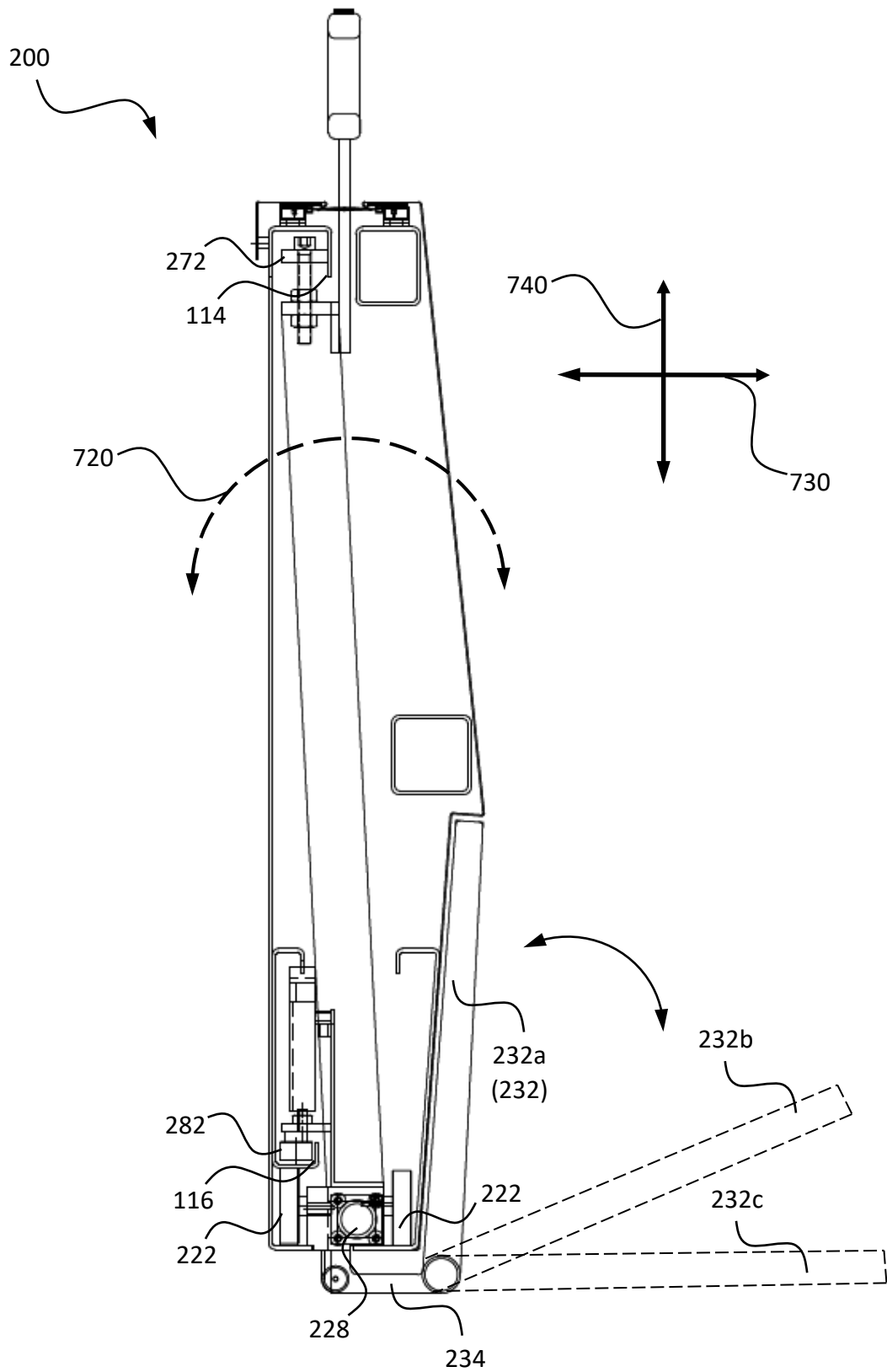
Fig. 6 (VIEW A-A)
