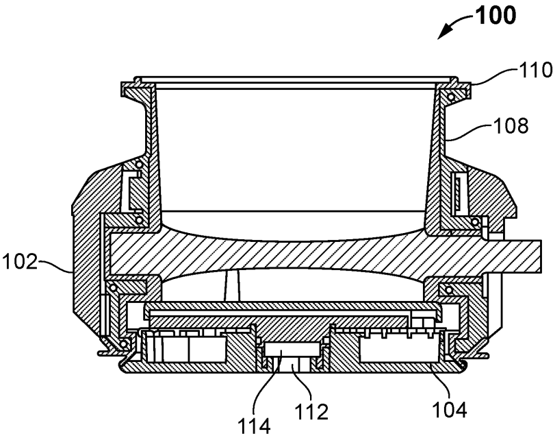
SECTION L-L FIG. 6B
