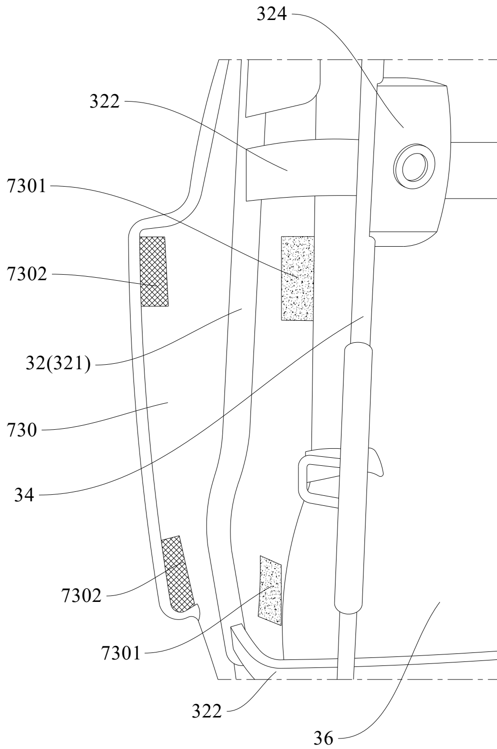
FIG. 55
